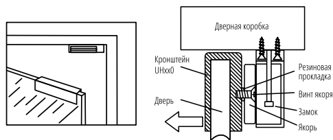
Рис. 4 Монтаж на стеклянную дверь с помощью кронштейна U типа (UHx0)
