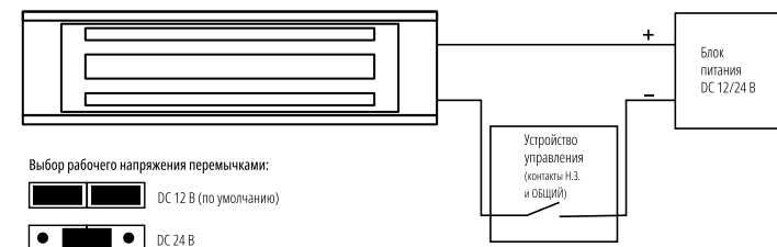
Рис. 10 Схема подключения DL280 и DL350
