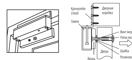
Рис. 2 Монтаж с помощью кронштейна L типа (LHxx0)
