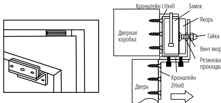
Рис. 3 Монтаж с помощью кронштейнов L и Z типов (LHx0, ZHx0)
