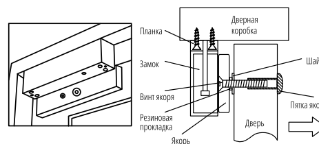
Рис. 1 Стандартный монтаж на дверную коробку
